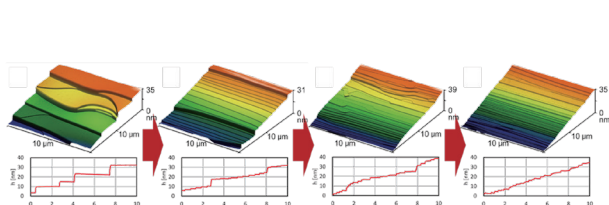
図1 SiCをAr/H 2 中で1600℃で加熱後してステップが高くなった後に、1400℃で保持した際の変化
