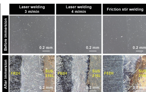
図2 CBB試験前後の異材継手表面観察結果
