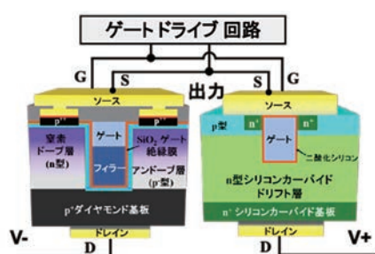
図1 ダイヤモンドp-FETとSiC n-FETによる相補型インバータ回路のハーフブリッジ。ソースが共通で出力。
