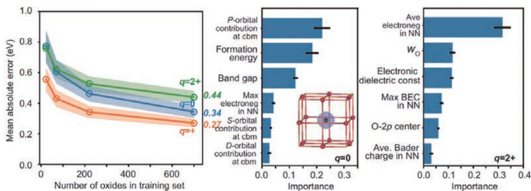
図1 第一原理計算データの機械学習による酸化物の酸素空孔形成エネルギーの予測モデル構築 [Y. Kumagai et al., Phys. Rev. Materials 5, 123803 (2021).]
