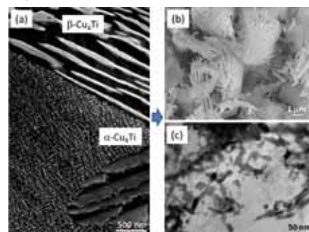
図1 (a) 時効処理したCu-4 wt.% Ti合金の組織。(b) (c) 抽出分離により採取した粗大 \beta -Cu 4 Tiおよび微細 \alpha -Cu 4 Ti析出物。
