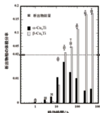
図2 450°C等温時効によるCu-4 at.% Ti合金中での析出物生成の推移。
