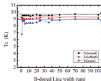
図2 超伝導転移温度の加工線幅依存性
